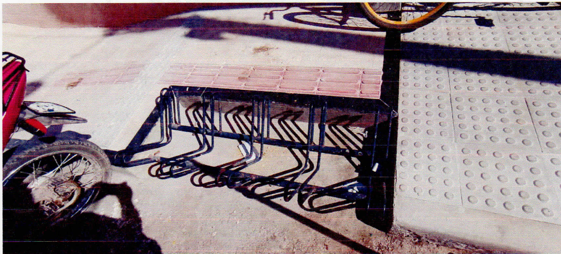
FOTO 04 –ASSENTAMENTO DE BICICLETÁRIO
